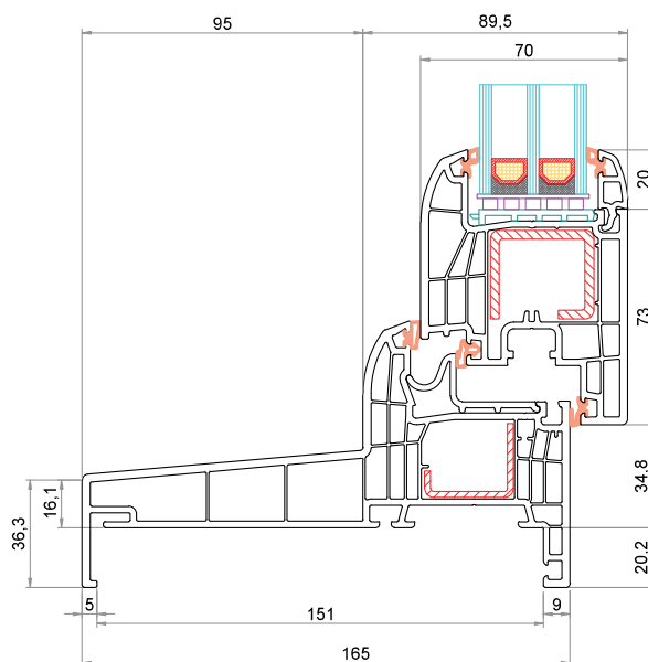
Telaio "Monoblocco" 165 mm CK-L028 Anta CK-Z041
