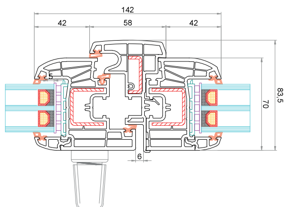
Anta CK-Z044 Battente mobile 58 mm CK-T046 Anta CK-Z044
