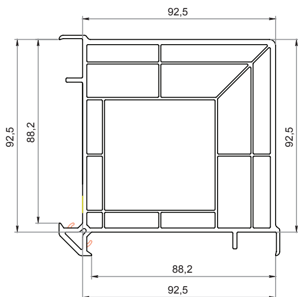
Connettore 90° 8355
