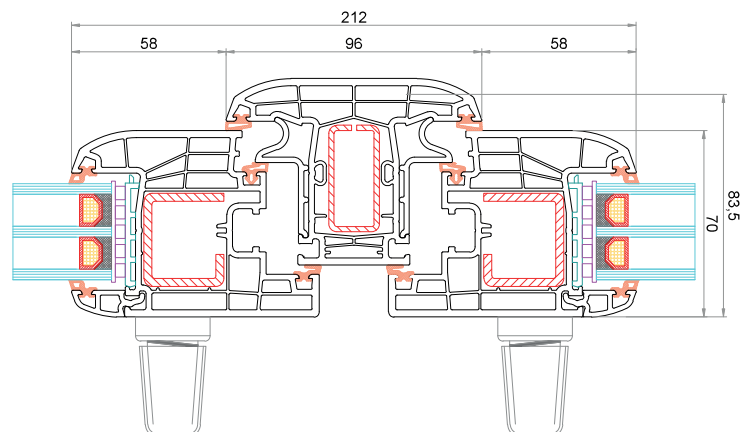
Anta CK-Z041 Montante fisso da 96 mm CK-T004 Anta CK-Z041
