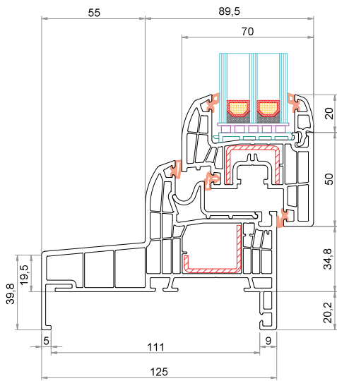
Telaio "Monoblocco" 125 mm CK-L026 Anta CK-Z043
