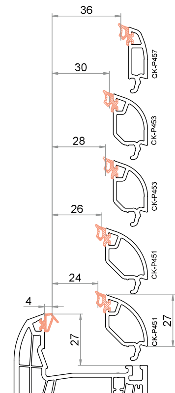
Telaio / Montante altezza della battuta 27 mm / altezza del fermavetro 27 mm
