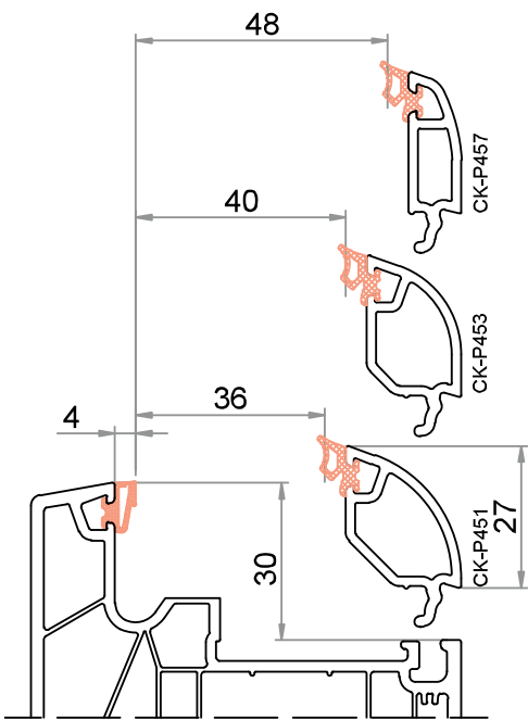
Telaio / Montante altezza della battuta 27 mm / altezza del fermavetro 27 mm
