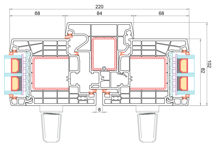
Anta CK-Z841 Profilo di copertura squadrato per maniglia centrale 76833 Battente mobile 64 mm CK-T864 Anta CK-Z841
