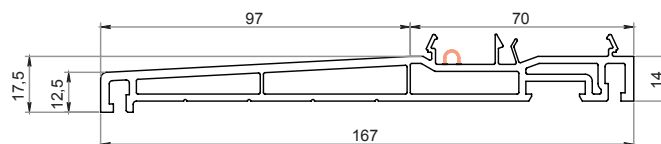
Davanzale 97 mm 6135
