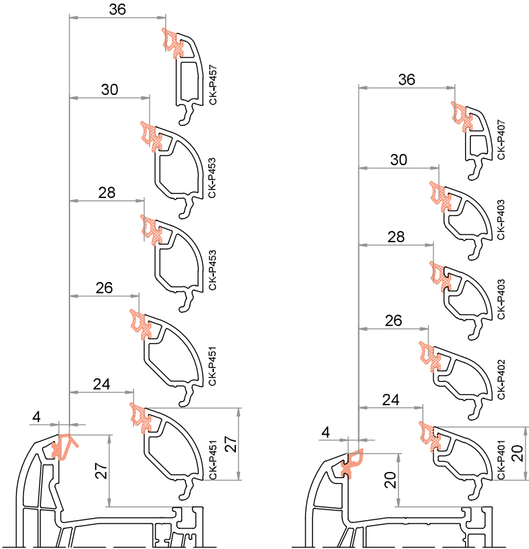
Telaio / Montante altezza della battuta 27 mm / altezza del fermavetro 27 mm
