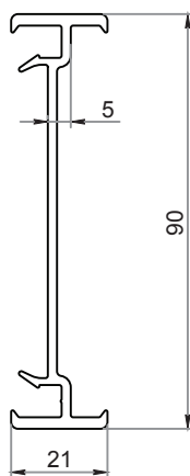
Connettore MINI 5 mm CK-E805
