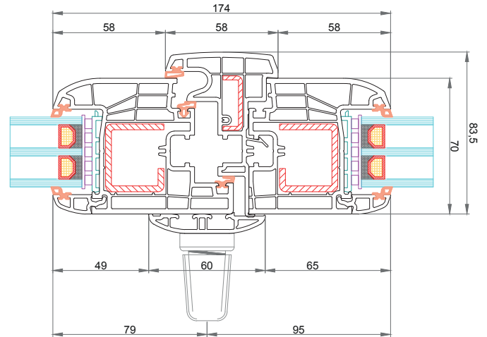
Anta CK-Z041 Profilo di copertura arrotondato per maniglia centrale CK-E036 Battente mobile 58 mm CK-T046 Anta CK-Z041
