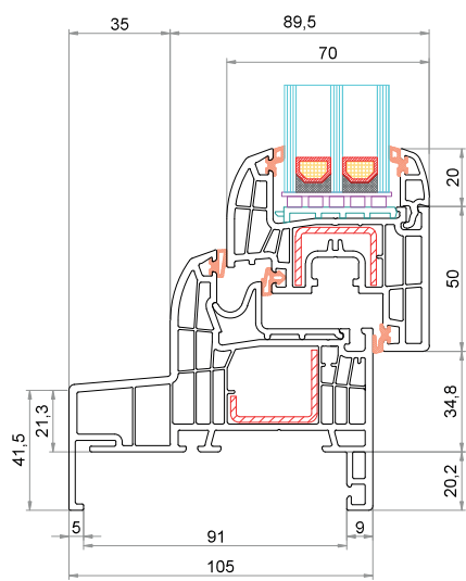
Telaio "Monoblocco" 105 mm CK-L025 Anta CK-Z043
