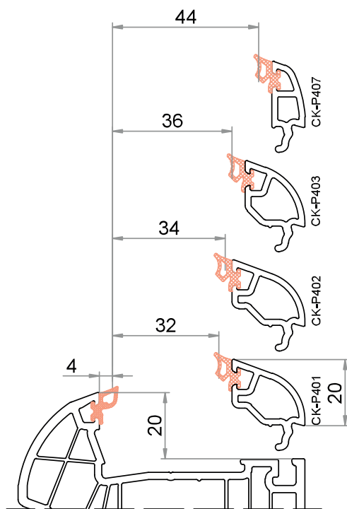
Anta / Traverso altezza della battuta 20 mm / altezza del fermavetro 20 mm
