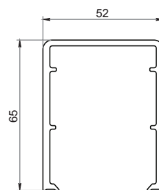
Profilo esterno di supporto 154
