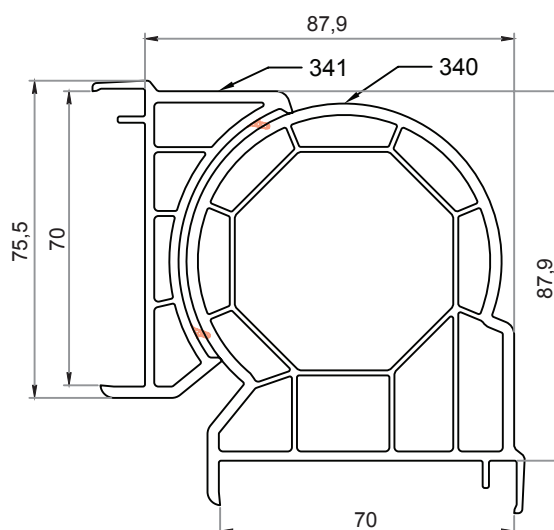
Connettore tubolare 340 + 341
