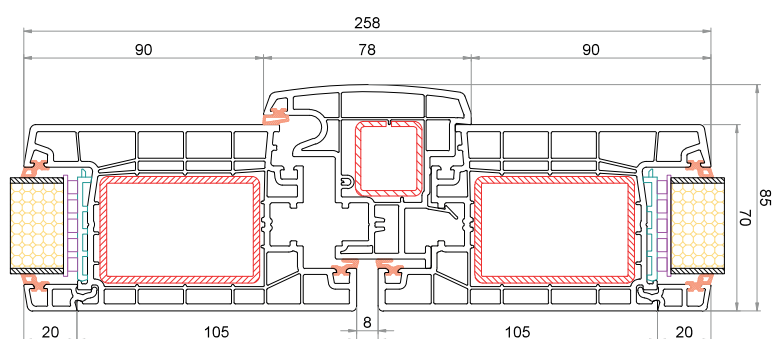
Anta CK-Z057 Battente mobile 78 mm CK-T045 Anta CK-Z057
