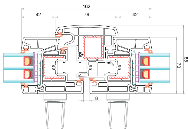
Anta CK-Z051 Battente mobile 78 mm CK-T045 Anta CK-Z051 (maniglia anche sull'anta secondaria)
