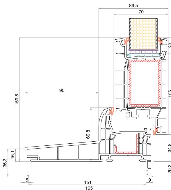
Telaio "Monoblocco" 165 mm CK-L028 Anta CK-Z057
