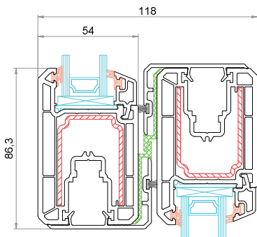
Anta 6041 Profilo di chiusura 6060 Anta 6041
