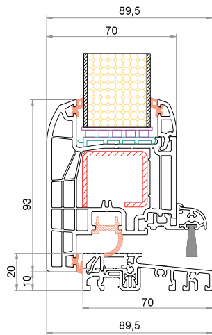
Anta CK-Z040 Soglia bassa 6-37852-60-0-1
