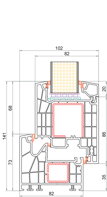
Telaio CK-L0802 Anta CK-Z841
