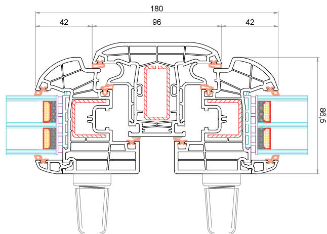
Anta CK-Z003 Montante fisso da 96 mm CK-T004 Anta CK-Z003
