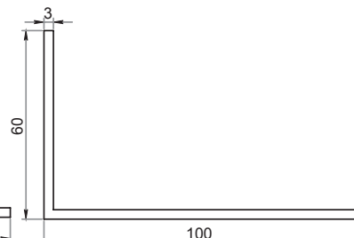
Barra angolare 60x100 mm 30C60100
