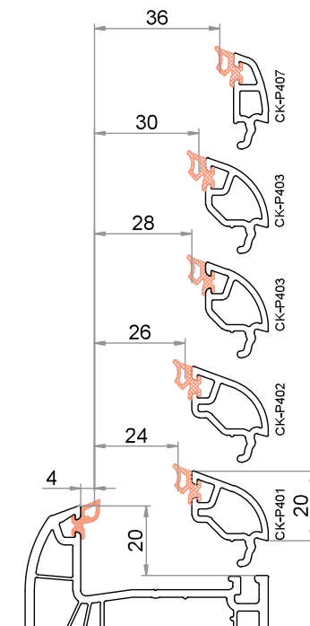
Anta / Traverso altezza della battuta 20 mm / altezza del fermavetro 20 mm
