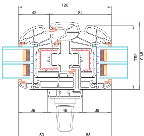
Anta CK-Z003 Profilo di copertura squadrato per maniglia centrale 76833 Anta - montante mobile 84 mm CK-Z030
