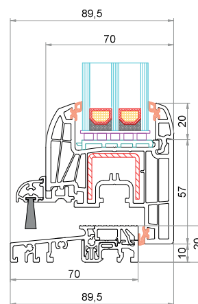
Anta CK-Z044 Soglia bassa 6-37852-60-0-1
