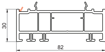
Allargatore da 30 mm CK-E881
