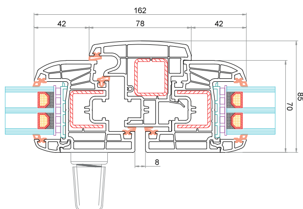
Anta CK-Z044 Battente mobile 78 mm CK-T045 Anta CK-Z044
