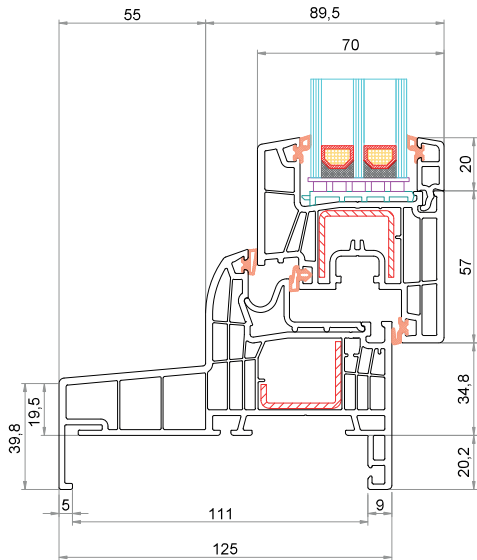
Telaio "Monoblocco" 125 mm CK-L026 Anta CK-Z051
