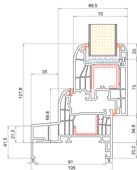
Telaio "Monoblocco" 105 mm CK-L025 Anta CK-Z041
