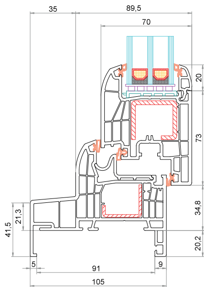
Telaio "Monoblocco" 105 mm CK-L025 Anta CK-Z041
