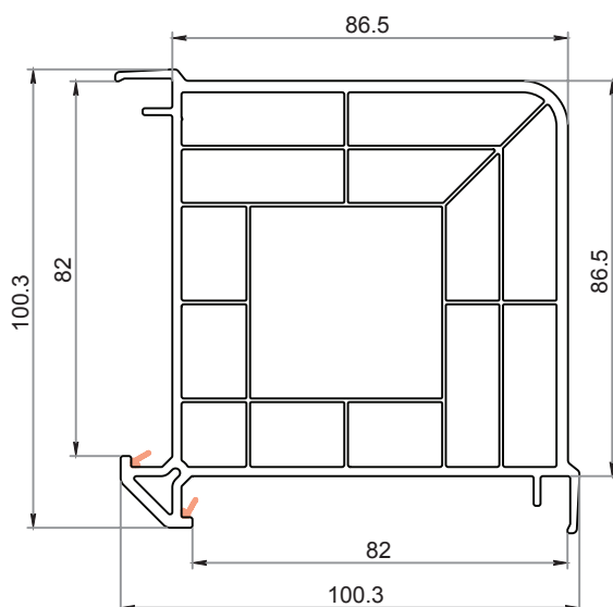
Connettore 90° CK-E890
