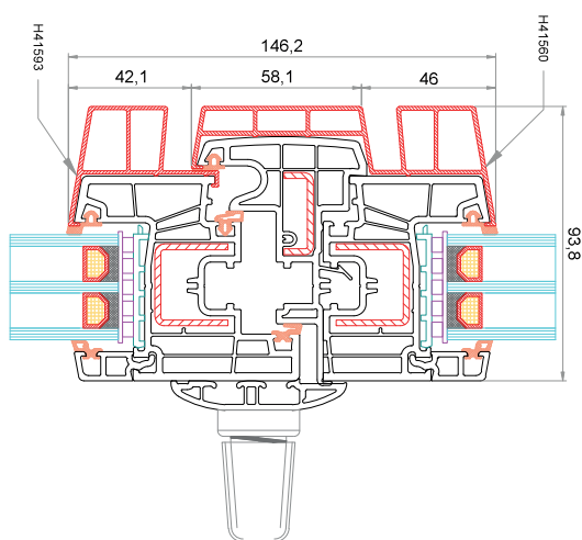
Anta CK-Z051 + AluClip H41593 Profilo di copertura arrotondato per maniglia centrale CK-E036 Battente mobile 58 mm CK-T046 Anta CK-Z051 + AluClip H41560
