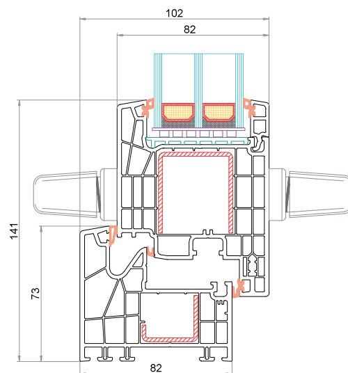
Telaio CK-L0802 Anta CK-Z841 (maniglia passante)
