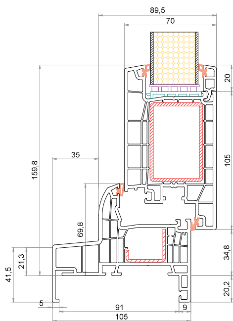
Telaio "Monoblocco" 105 mm CK-L025 Anta CK-Z057
