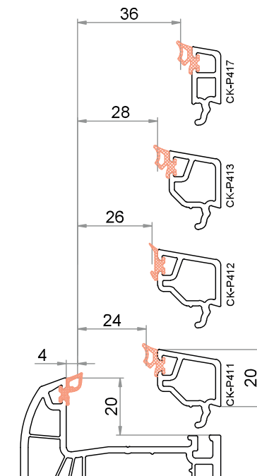
Anta / Trasverso altezza della battuta 20 mm / altezza del fermavetro 20 mm
