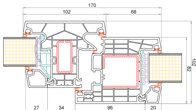
Anta CK-Z841 Montante fisso da 96 mm CK-T803
