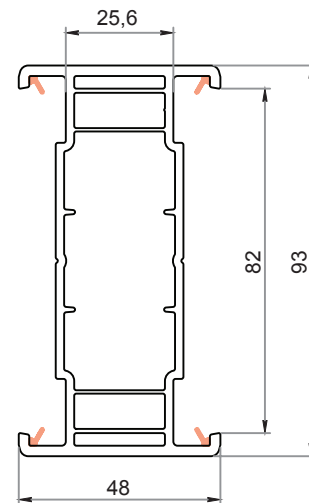
Connettore statico 30 mm CK-E880
