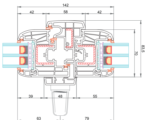
Anta CK-Z044 Profilo di copertura squadrato per maniglia centrale 76833 Battente mobile 58 mm CK-T046 Anta CK-Z044
