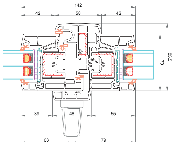
Anta CK-Z051 Profilo di copertura squadro per maniglia centrale 76833 Battente mobile 58 mm CK-T046 Anta CK-Z051
