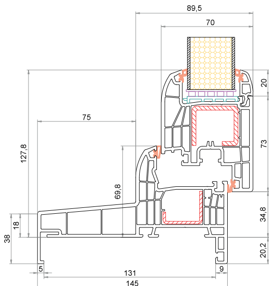
Telaio "Monoblocco" 145 mm CK-L027 Anta CK-Z041
