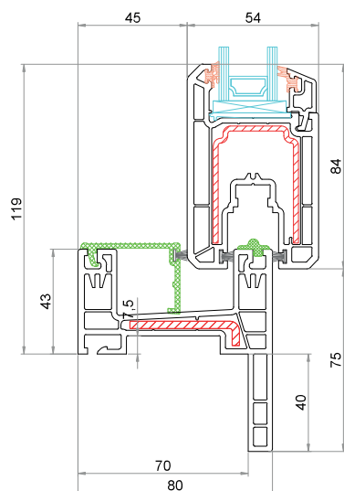
Telaio Reno 40 mm 6051 Anta 6041 Tappo per parte fissa 9C62
