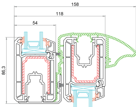
Anta 6041 Profilo di chiusura 9C58 Anta 6041
