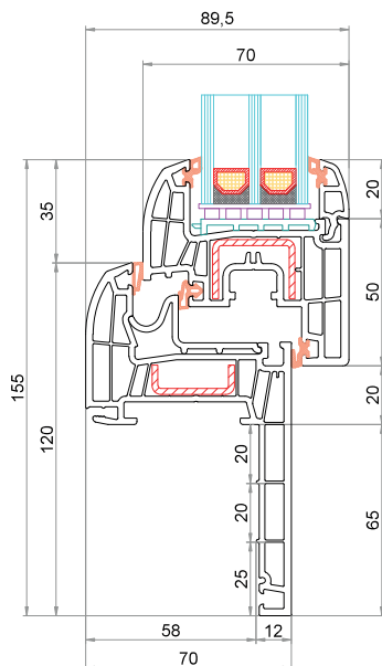
Telaio Reno 65 mm CK-L065 Anta CK-Z043
