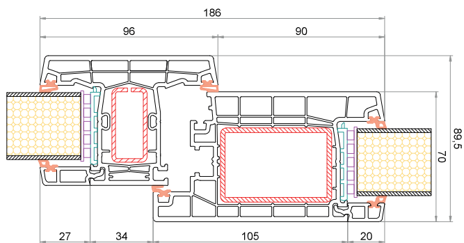
Anta CK-Z057 Montante fisso da 96 mm CK-T050
