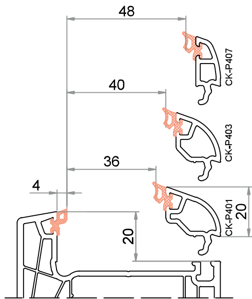
Anta / Traverso altezza della battuta 20 mm / altezza del fermavetro 20 mm
