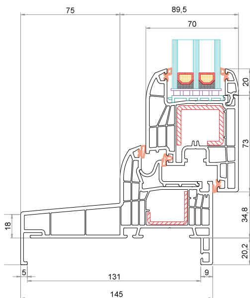
Telaio "Monoblocco" 145 mm CK-L027 Anta CK-Z041
