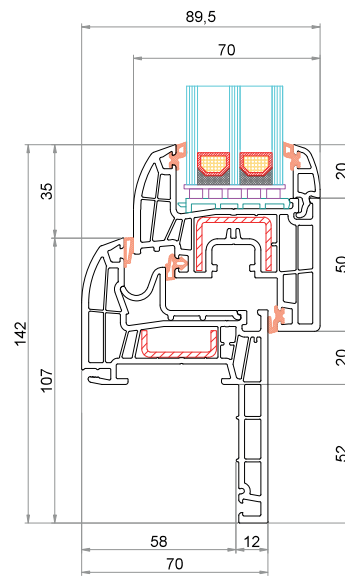
Anta CK-Z043 Soglia bassa 6-37852-60-0-1
