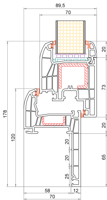
Telaio Reno 65 mm CK-L065 Anta CK-Z041
