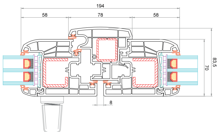
Anta CK-Z041 Battente mobile 78 mm CK-T045 Anta CK-Z041
