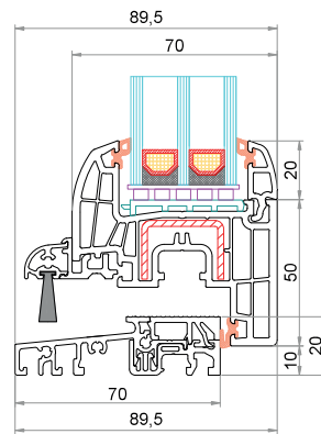
Anta CK-Z043 Soglia bassa 6-37852-60-0-1
