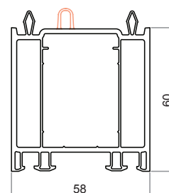
Allargatore da 60 mm 546
