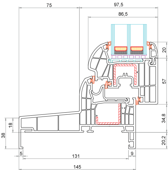
Telaio "Monoblocco" 145 mm CK-L027 Anta CK-Z003
