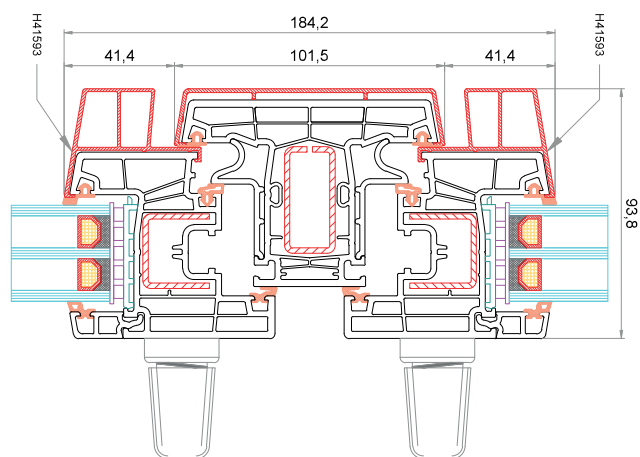
Anta CK-Z051 + AluClip H41593 Montante fisso da 96 mm CK-T050 + AluClip F53674 Anta CK-Z051 + AluClip H41593
