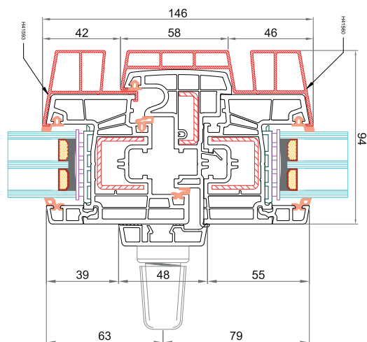
Anta CK-Z051 + AluClip H41593 Profilo di copertura squadrato per maniglia centrale 76833 Battente mobile 58 mm CK-T046 Anta CK-Z051 + AluClip H41560
