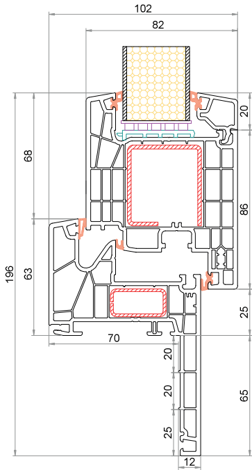
Telaio Reno 65 mm CK-L0865 Anta CK-Z841
