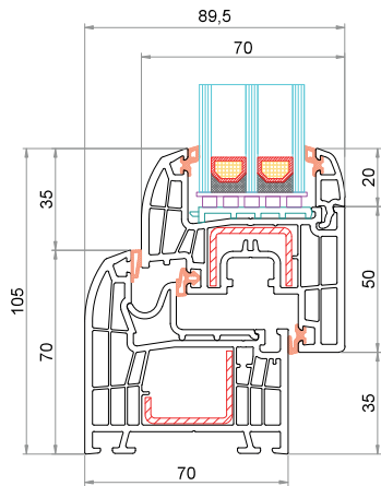
Telaio CK-L001 Anta CK-Z043
