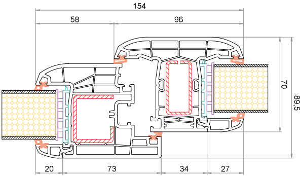
Anta CK-Z041 Montante fisso da 96 mm CK-T004
