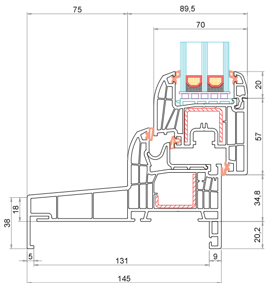
Telaio "Monoblocco" 145 mm CK-L027 Anta CK-Z044
