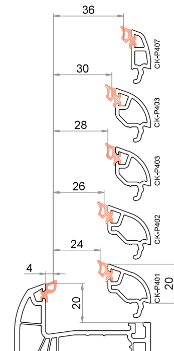
Anta / Trasverso altezza della battuta 20 mm / altezza del fermavetro 20 mm
