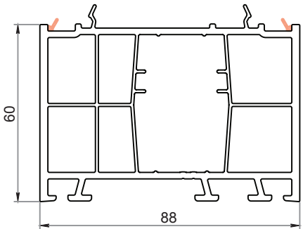
Allargatore da 60 mm CK-E106
