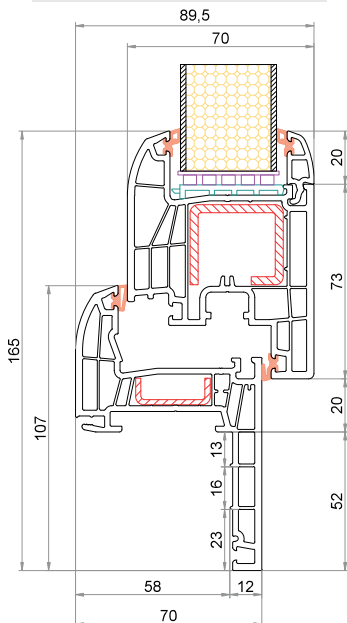
Telaio Reno 52 mm CK-L029 Anta CK-Z041
