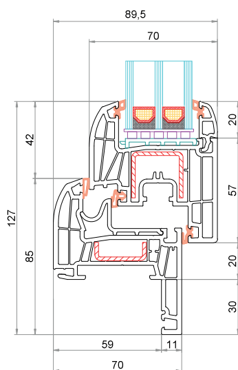
Telaio Reno 30 mm CK-L031 Anta CK-Z044
