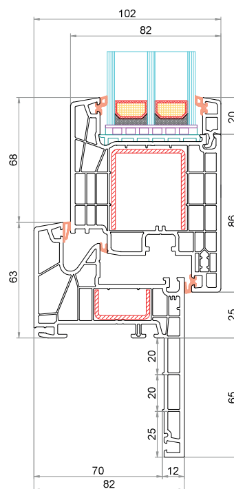
Telaio Reno 65 mm CK-L0865 Anta CK-Z841
