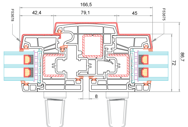
Anta CK-Z051 + AluClip F53678 Battente mobile 78 mm CK-T045 Anta CK-Z051 (maniglia anche sull'anta secondaria) + AluClip F53675
