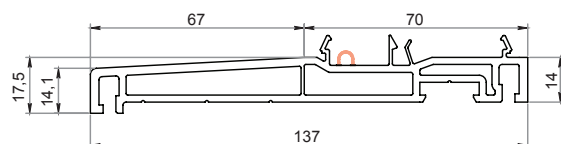
Davanzale 67 mm 6134
