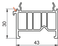
Listello sotto davanzale / da trasporto 30 mm CK-E100
