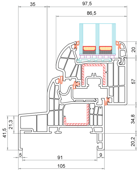
Telaio "Monoblocco" 105 mm CK-L025 Anta CK-Z003
