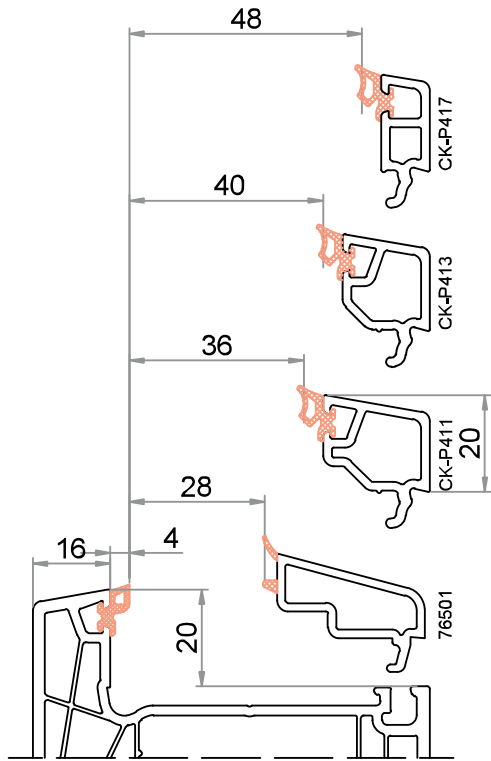
Anta / Traverso altezza della battuta 20 mm / altezza del fermavetro 20 mm
