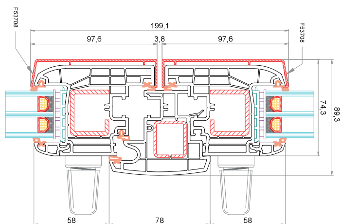
Anta CK-Z040 + AluClip F53708 Battente mobile 78 mm CK-T045 Anta CK-Z040 (maniglia anche sull'anta secondaria) + AluClip F53708
