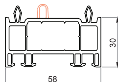
Allargatore da 30 mm 144
