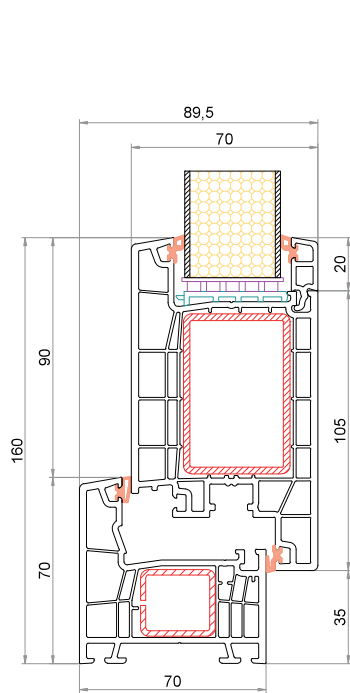
Telaio CK-L052 Anta CK-Z057
