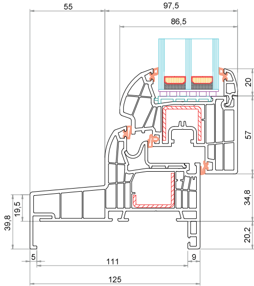
Telaio "Monoblocco" 125 mm CK-L026 Anta CK-Z003
