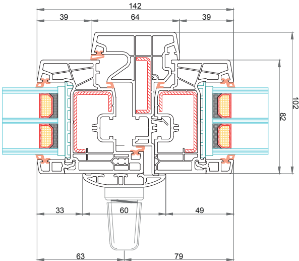
Anta CK-Z801 Profilo di copertura arrotondato per maniglia centrale CK-E036 Battente mobile 64 mm CK-T864 Anta CK-Z801
