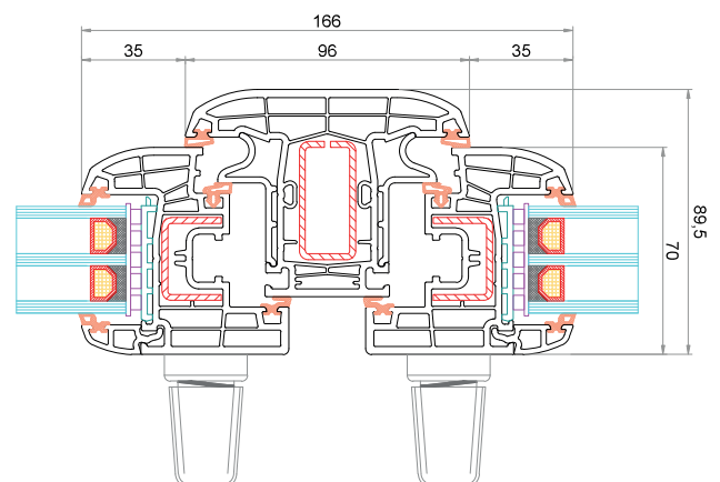
Anta CK-Z043 Montante fisso da 96 mm CK-T004 Anta CK-Z043
