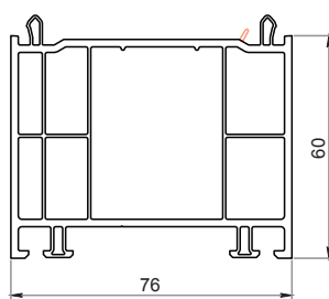
Allargatore da 60 mm 76702
