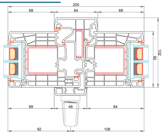
Anta CK-Z841 Profilo di copertura squadrato per maniglia centrale 76833 Battente mobile 64 mm CK-T864 Anta CK-Z841
