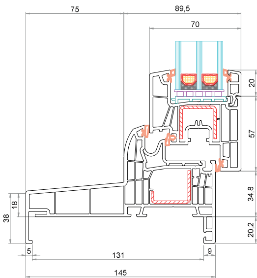
Telaio "Monoblocco" 145 mm CK-L027 Anta CK-Z051
