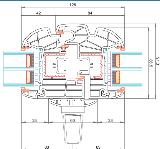
Anta CK-Z003 Profilo di copertura arrotondato per maniglia centrale CK-E036 Anta - montante mobile 84 mm CK-Z030
