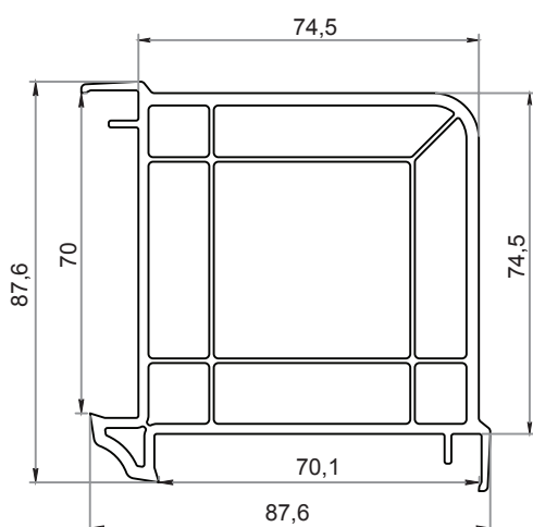
Connettore 90° 355
