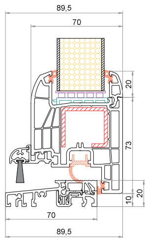
Anta CK-Z041 Soglia bassa 6-37852-60-0-1
