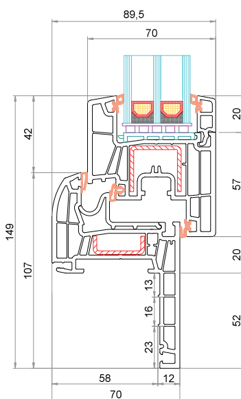
Telaio Reno 52 mm CK-L029 Anta CK-Z051
