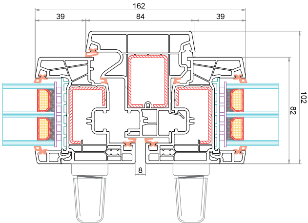
Anta CK-Z801 Profilo di copertura squadrato per maniglia centrale 76833 Battente mobile 64 mm CK-T864 Anta CK-Z801
