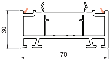
Allargatore da 30 mm CK-E081
