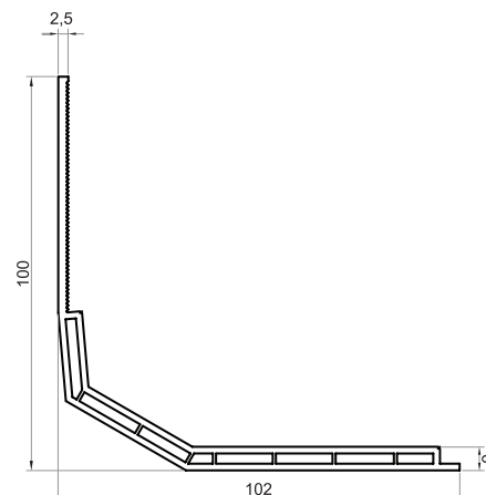
Barra angolare scatolato 100x100 mm PA10010025
