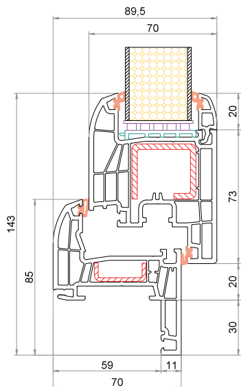
Telaio Reno 30 mm CK-L031 Anta CK-Z041
