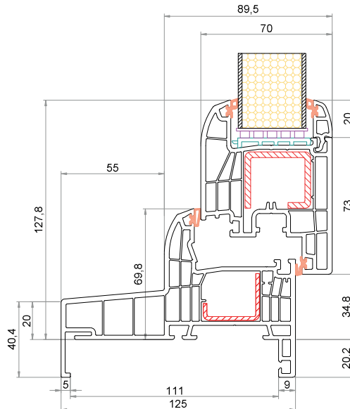
Telaio "Monoblocco" 125 mm CK-L026 Anta CK-Z041
