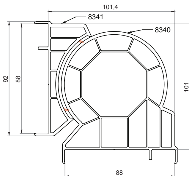
Connettore tubolare 8340 + 8341
