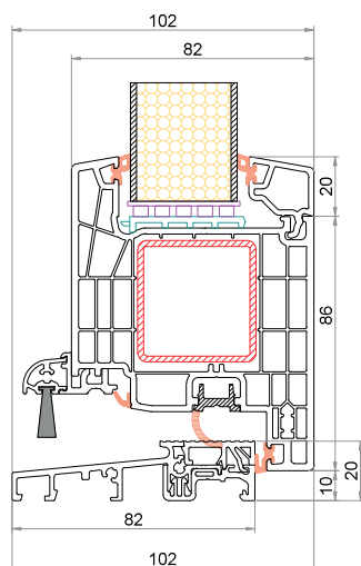
Anta CK-Z841 Soglia bassa 6-37479-60-0-1
