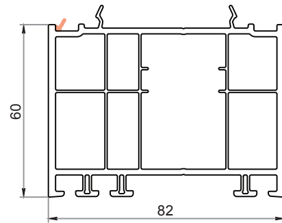
Allargatore da 60 mm CK-E882
