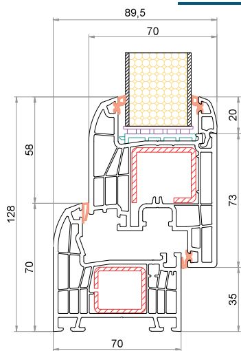
Telaio CK-L001 Anta CK-Z041
