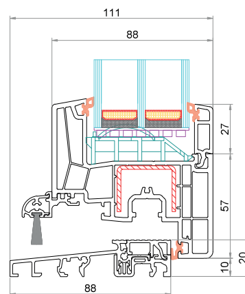
Anta CK-Z101 Soglia bassa 6-338967-99-0-00
