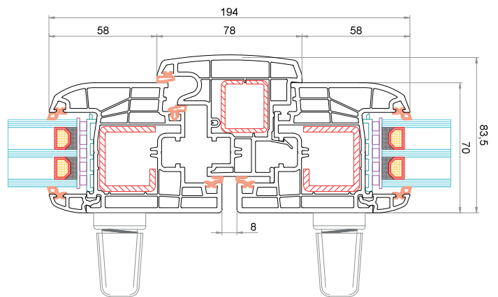
Anta CK-Z041 Battente mobile 78 mm CK-T045 Anta CK-Z041 (maniglia anche sull'anta secondaria)
