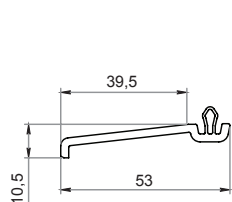
Davanzale 39.5 mm 76759
