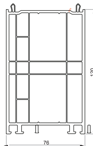
Allargatore da 120 mm 76703
