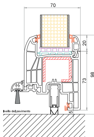
Anta CK-Z041 Barra parafreddo (nessuna soglia bassa)
