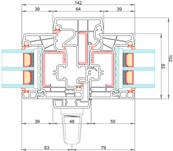
Anta CK-Z801 Profilo di copertura squadrato per maniglia centrale 76833 Battente mobile 64 mm CK-T864 Anta CK-Z801
