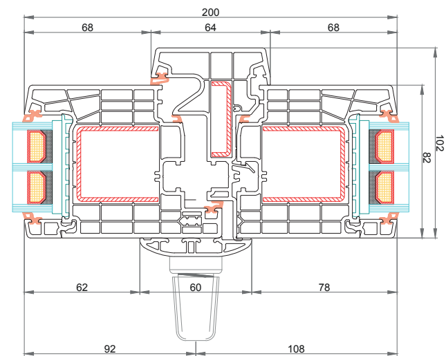
Anta CK-Z841 Profilo di copertura arrotondato per maniglia centrale CK-E036 Battente mobile 64 mm CK-T864 Anta CK-Z841
