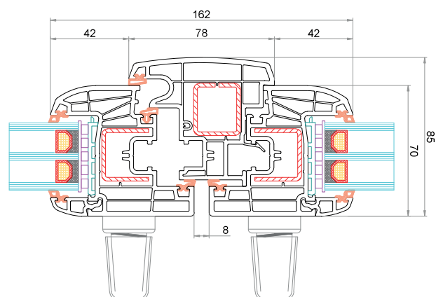
Anta CK-Z044 Battente mobile 78 mm CK-T045 Anta CK-Z044 (maniglia anche sull'anta secondaria)
