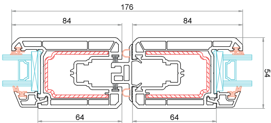
Anta 6041 Battente mobile 6067 Anta 6041
