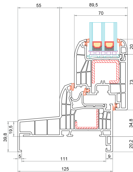
Telaio "Monoblocco" 125 mm CK-L026 Anta CK-Z041
