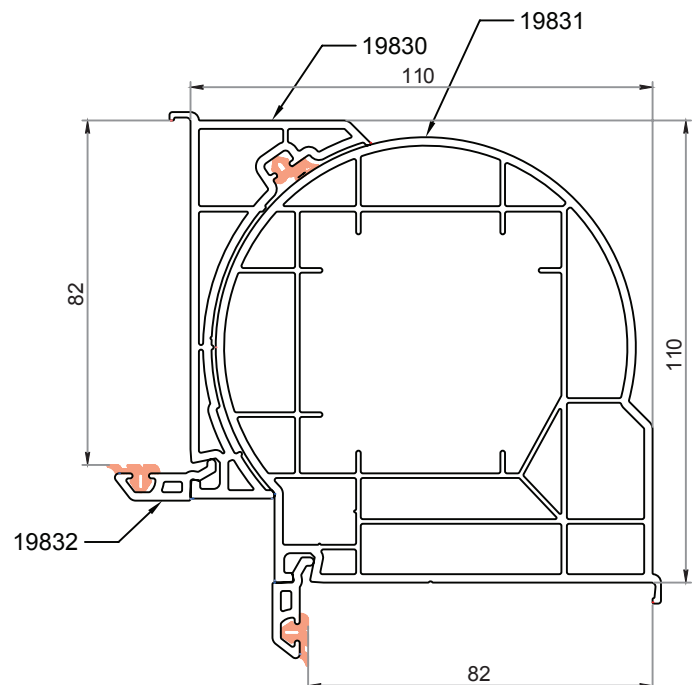
Connettore tubolare 19830 + 19831 + 19832
