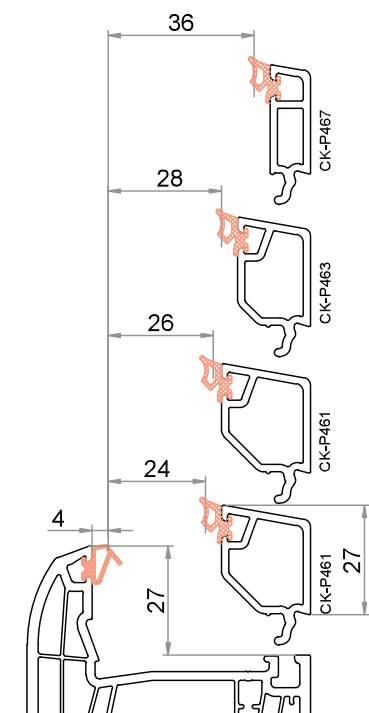
Telaio / Montante altezza della battuta 27 mm / altezza del fermavetro 27 mm
