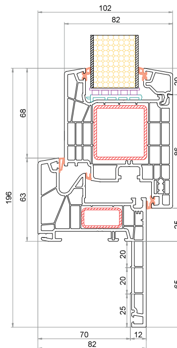
Telaio Reno 65 mm CK-L0865 Anta CK-Z841
