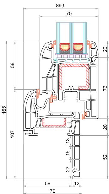
Telaio Reno 52 mm CK-L029 Anta CK-Z041
