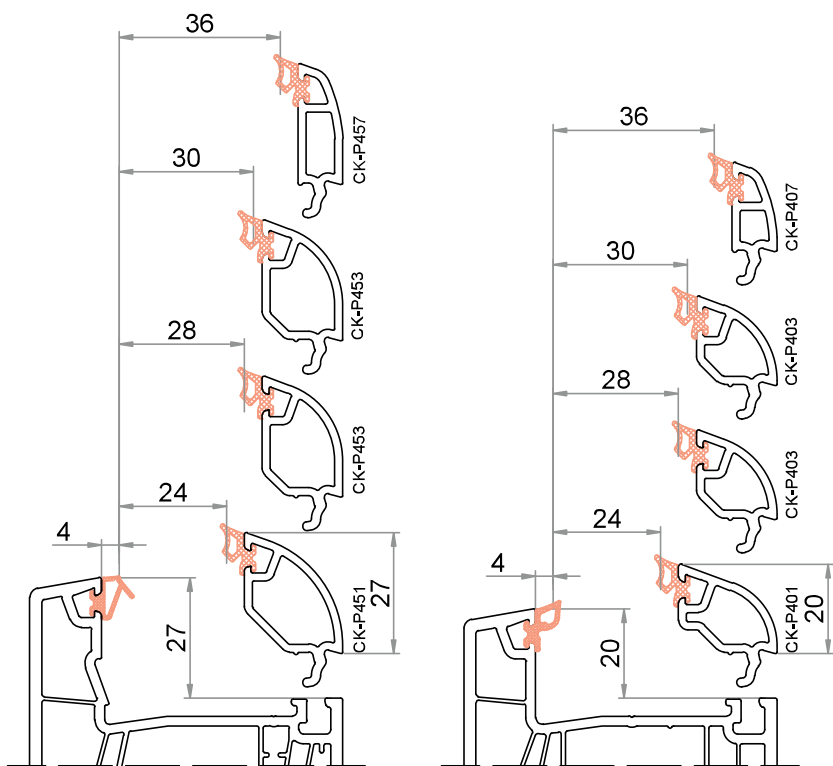
Telaio / Montante altezza della battuta 27 mm / altezza del fermavetro 27 mm
