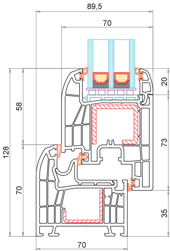
Telaio CK-L001 Anta CK-Z041
