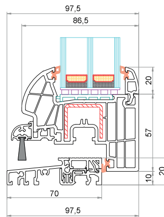
Anta CK-Z003 Soglia bassa 6-37852-60-0-1
