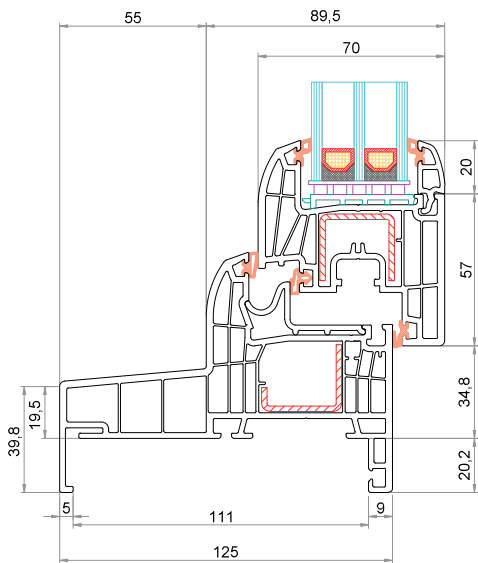
Telaio "Monoblocco" 125 mm CK-L026 Anta CK-Z044
