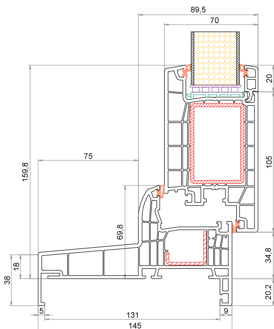
Telaio "Monoblocco" 145 mm CK-L027 Anta CK-Z057
