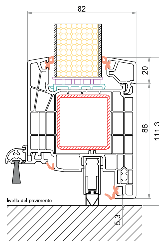
Anta CK-Z841 Barra parafreddo (nessuna soglia bassa)
