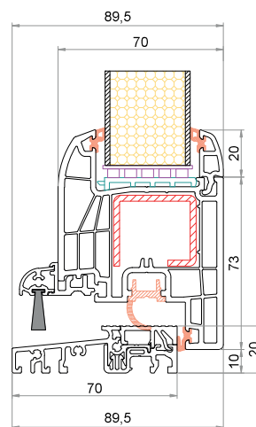
Anta CK-Z041 Soglia bassa 6-37852-60-0-1
