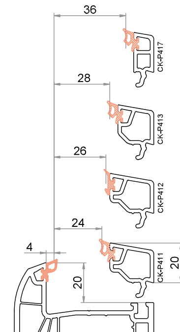
Anta / Traverso altezza della battuta 20 mm / altezza del fermavetro 20 mm
