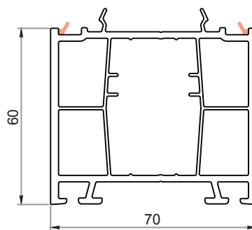
Allargatore da 60 mm CK-E082
