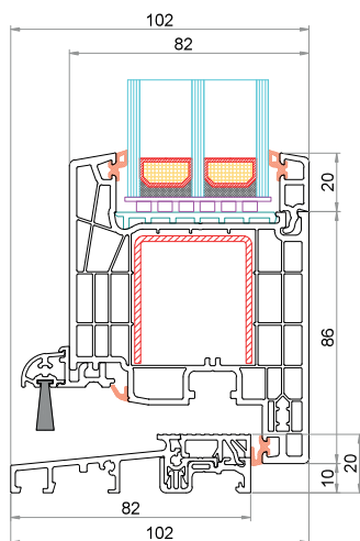
Anta CK-Z841 Soglia bassa 6-37479-60-0-1
