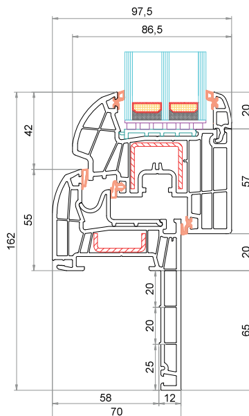
Telaio Reno 65 mm CK-L065 Anta CK-Z003
