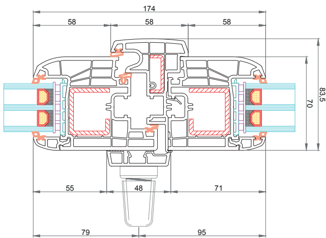
Anta CK-Z041 Profilo di copertura squadrato per maniglia centrale 76833 Battente mobile 58 mm CK-T046 Anta CK-Z041
