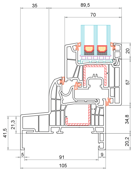
Telaio "Monoblocco" 105 mm CK-L025 Anta CK-Z051
