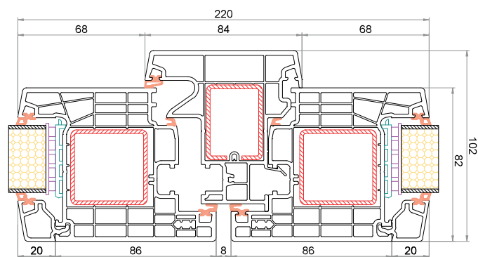
Anta CK-Z841 Battente mobile 84 mm CK-T884 Anta CK-Z841
