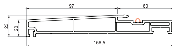
Davanzale 97 mm 6137
