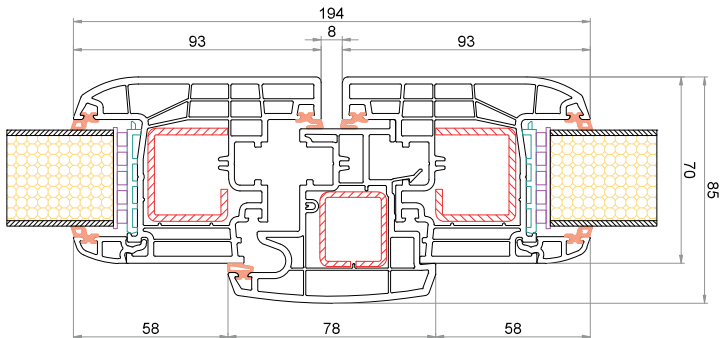
Anta CK-Z040 Battente mobile 78 mm CK-T045 Anta CK-Z040
