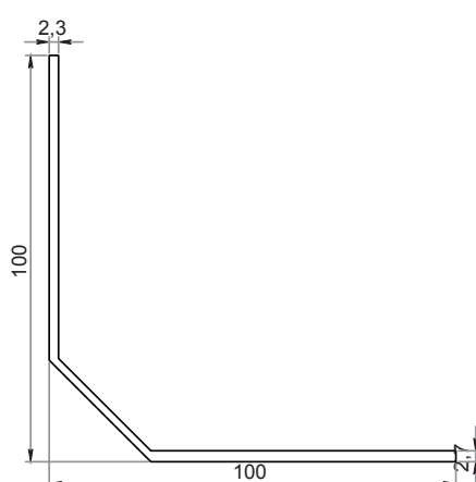
Barra angolare con angolo smussato 75x25x75 mm C752575
