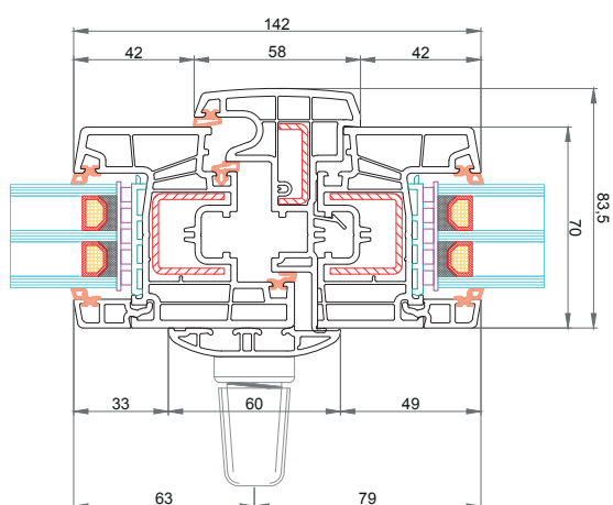
Anta CK-Z051 Profilo di copertura arrotondato per maniglia centrale CK-E036 Battente mobile 58 mm CK-T046 Anta CK-Z051
