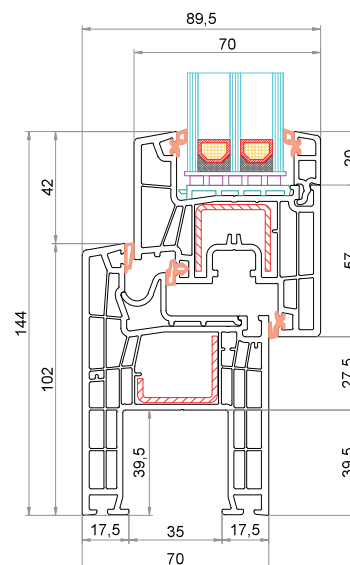
Telaio svizzero CK-L053 Anta CK-Z051
