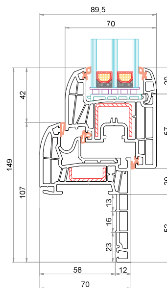
Telaio Reno 52 mm CK-L029 Anta CK-Z044
