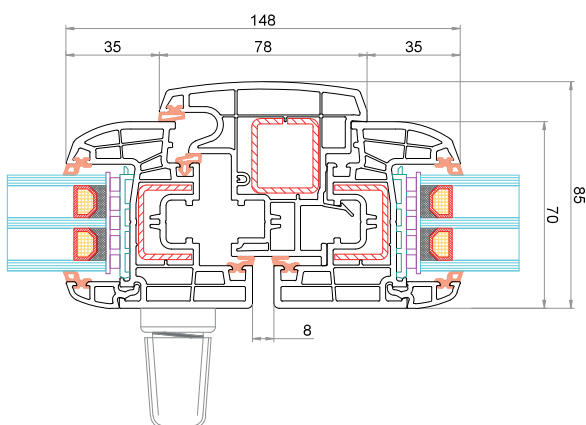
Anta CK-Z043 Battente mobile 78 mm CK-T045 Anta CK-Z043
