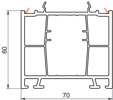
Allargatore da 60 mm CK-E082
