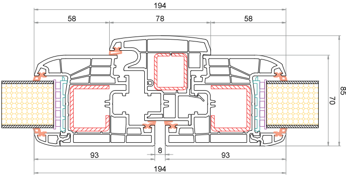
Anta CK-Z041 Battente mobile 78 mm CK-T045 Anta CK-Z041
