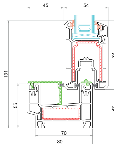
Telaio ristretto 6054 Anta 6041 Tappo per parte fissa 9C62
