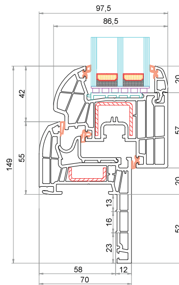
Anta CK-Z003 Soglia bassa 6-37852-60-0-1
