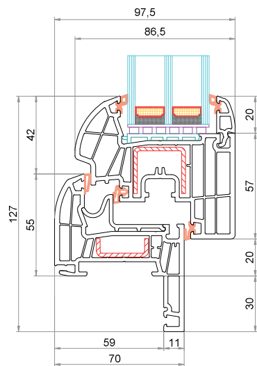
Telaio Reno 30 mm CK-L031 Anta CK-Z003
