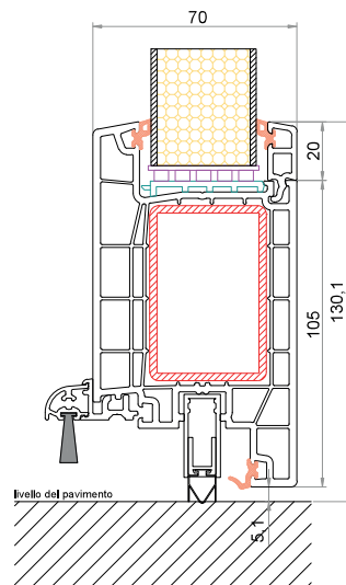
Anta CK-Z057 Barra parafreddo (nessuna soglia bassa)
