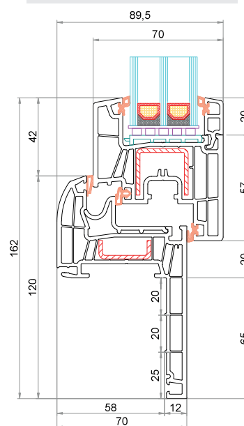
Telaio Reno 65 mm CK-L065 Anta CK-Z051
