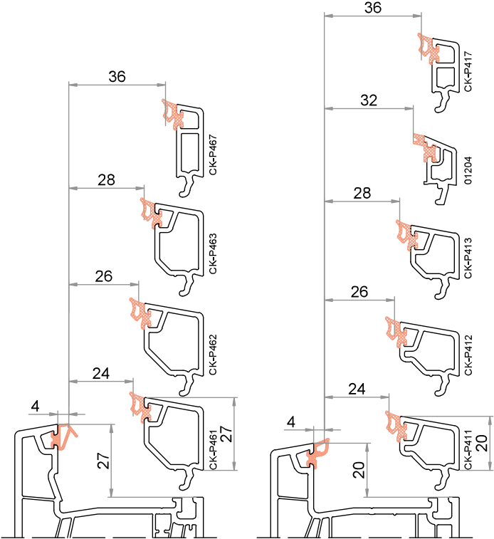
Telaio / Montante altezza della battuta 27 mm / altezza del fermavetro 27 mm
