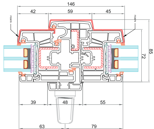
Anta CK-Z051 + AluClip F53678 Profilo di copertura squadrato per maniglia centrale 76833 Battente mobile 58 mm CK-T046 Anta CK-Z051 + AluClip F53679
