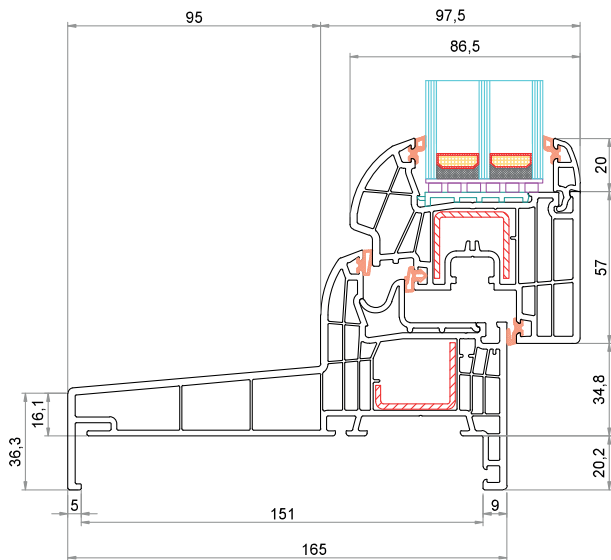
Telaio "Monoblocco" 165 mm CK-L028 Anta CK-Z003
