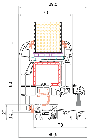
Anta CK-Z040 Soglia bassa 6-37852-60-0-1
