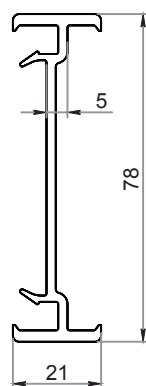
Connettore H 5 mm 350
