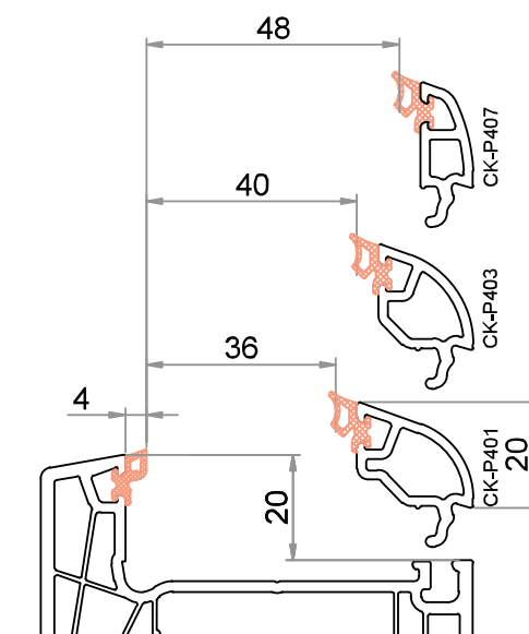
Anta / Traverso altezza della battuta 20 mm / altezza del fermavetro 20 mm
