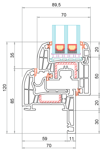
Telaio Reno 30 mm CK-L031 Anta CK-Z043
