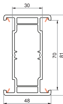
Connettore statico 30 mm CK-E080
