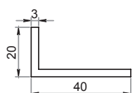
Barra angolare 20x40 mm 30C2040
