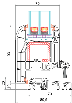
Anta CK-Z040 Soglia bassa 6-37852-60-0-1
