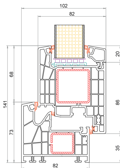
Telaio CK-L0802 Anta CK-Z841
