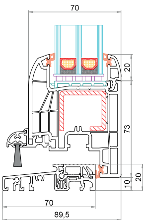
Anta CK-Z041 Soglia bassa 6-37852-60-0-1
