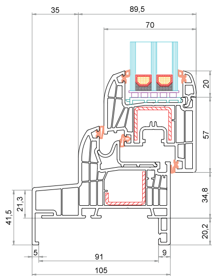
Telaio "Monoblocco" 105 mm CK-L025 Anta CK-Z044
