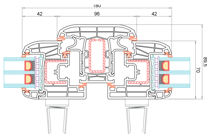
Anta CK-Z044 Montante fisso da 96 mm CK-T004 Anta CK-Z044
