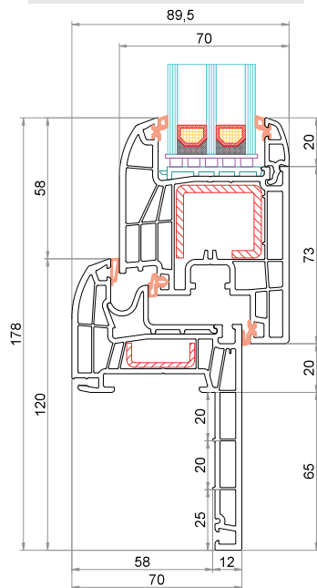
Telaio Reno 65 mm CK-L065 Anta CK-Z041
