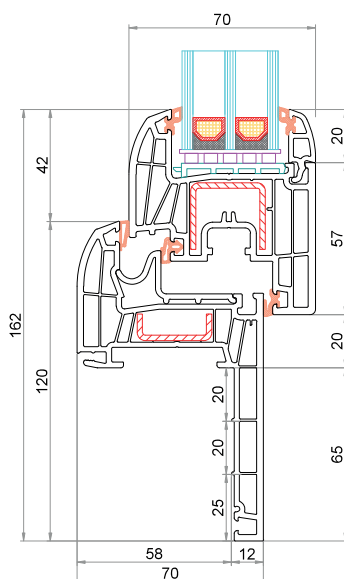
Telaio Reno 65 mm CK-L065 Anta CK-Z044
