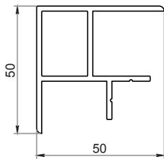
Angolare di chiusura CK-E304
