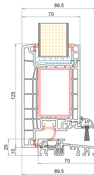
Anta CK-Z056 Soglia bassa 6-37852-60-0-1
