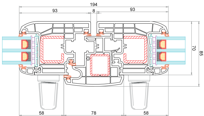
Anta CK-Z040 Battente mobile 78 mm CK-T045 Anta CK-Z040 (maniglia anche sull'anta secondaria)
