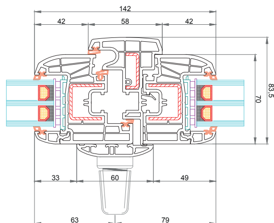
Anta CK-Z044 Profilo di copertura arrotondato per maniglia centrale CK-E036 Battente mobile 58 mm CK-T046 Anta CK-Z044
