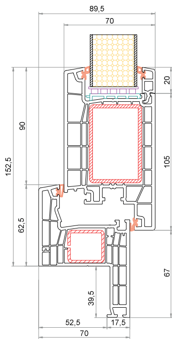
Telaio Reno 39,5 mm CK-L053R Anta CK-Z057
