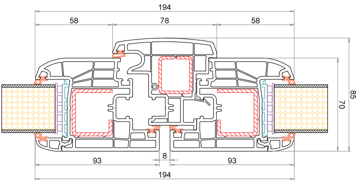
Anta CK-Z041 Battente mobile 78 mm CK-T045 Anta CK-Z041
