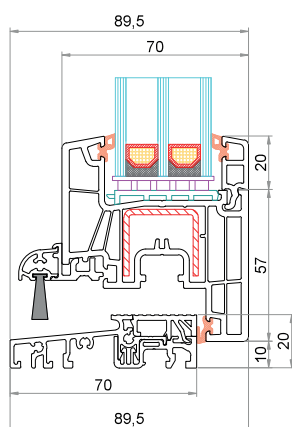
Anta CK-Z051 Soglia bassa 6-37852-60-0-1
