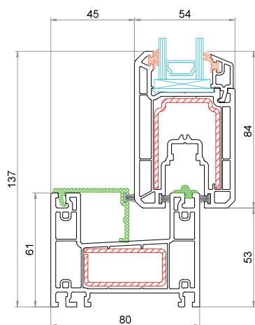
Telaio 6052 Anta 6041 Tappo per parte fissa 9C62
