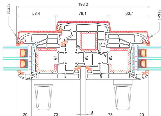
Anta CK-Z041 + AluClip F53706 Battente mobile 78 mm CK-T045 Anta CK-Z041 (maniglia anche sull'anta secondaria) + AluClip F54242
