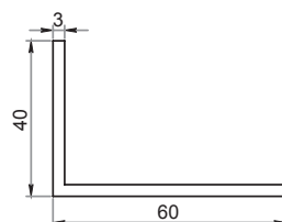
Barra angolare 40x60 mm 30C4060
