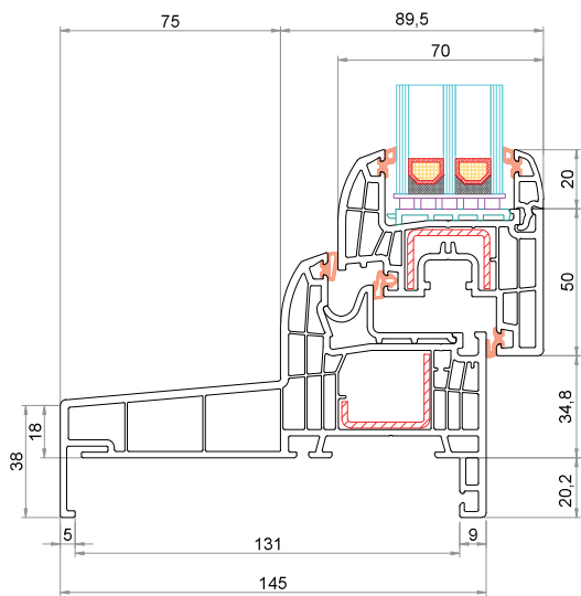
Telaio "Monoblocco" 145 mm CK-L027 Anta CK-Z043
