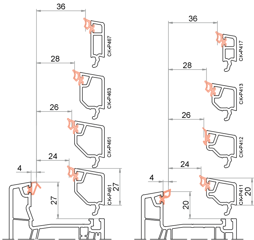
Telaio / Montante altezza della battuta 27 mm / altezza del fermavetro 27 mm
