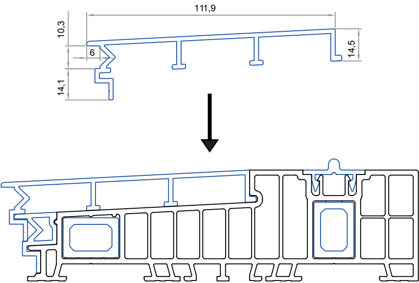
Profilo di comfort / Profilo supplementare CK-ALHS003
