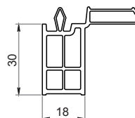
Allargatore da 30 mm 346
