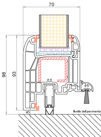
Anta CK-Z040 Barra parafreddo (nessuna soglia bassa)
