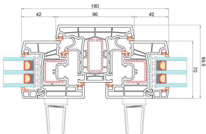
Anta CK-Z051 Montante fisso da 96 mm CK-T050 Anta CK-Z051
