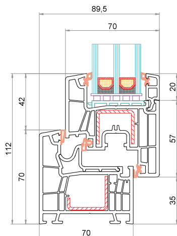
Telaio CK-L052 Anta CK-Z051
