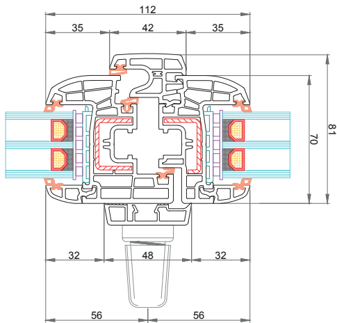
Anta CK-Z043 Profilo di copertura squadrato per maniglia centrale 76833 Battente mobile 42 mm CK-T037 Anta CK-Z043
