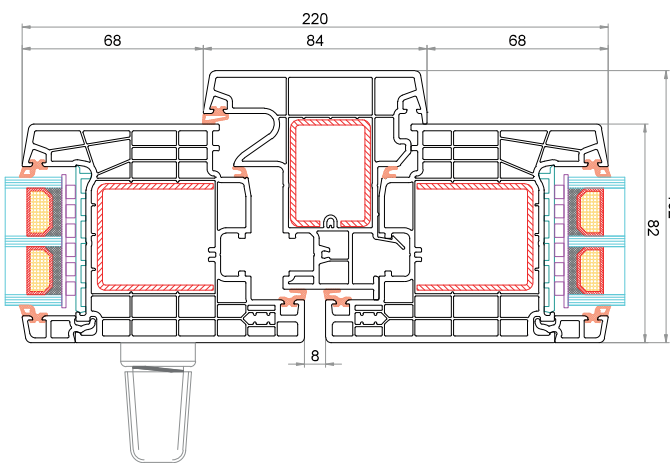
Anta CK-Z841 Battente mobile 84 mm CK-T884 Anta CK-Z841
