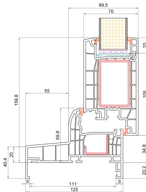
Telaio "Monoblocco" 125 mm CK-L026 Anta CK-Z057
