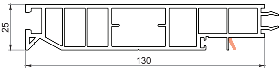
Parete del cassonetto/celino CK-E303
