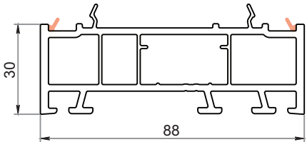
Allargatore da 30 mm CK-E105
