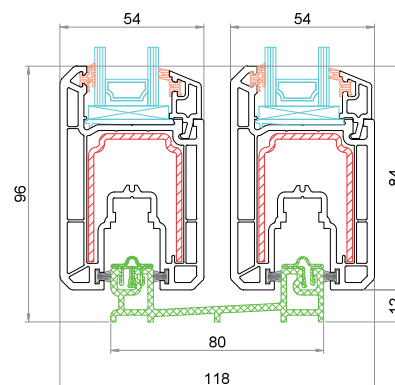
Anta 6041 Soglia bassa 9C66
