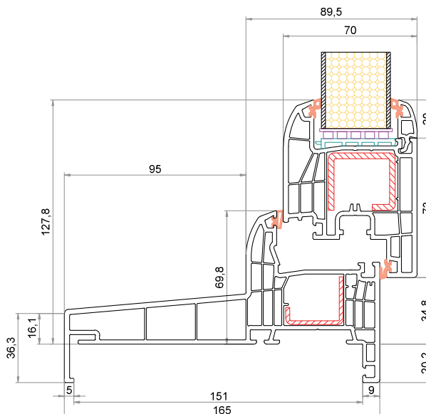
Telaio "Monoblocco" 165 mm CK-L028 Anta CK-Z041
