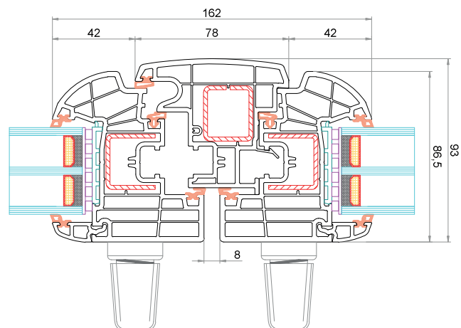
Anta CK-Z003 Battente mobile 78 mm CK-T045 Anta CK-Z003 (maniglia anche sull'anta secondaria)
