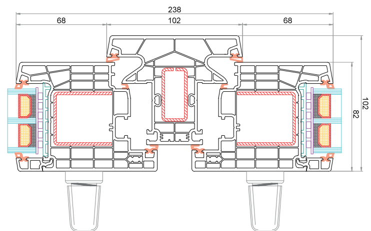
Anta CK-Z841 Montante fisso da 102 mm CK-T803 Anta CK-Z841
