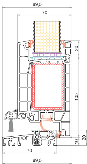
Anta CK-Z057 Soglia bassa 6-37852-60-0-1
