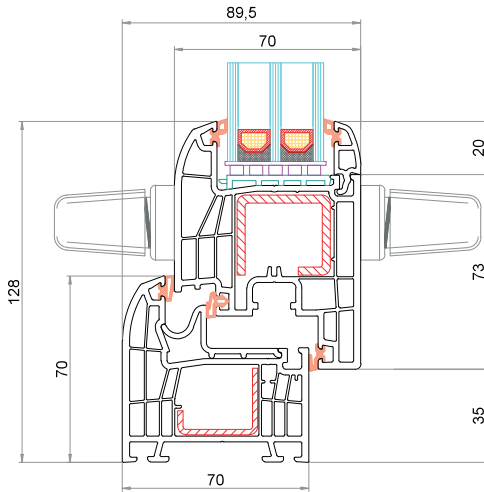
Telaio CK-L001 Anta CK-Z041 (maniglia passante)
