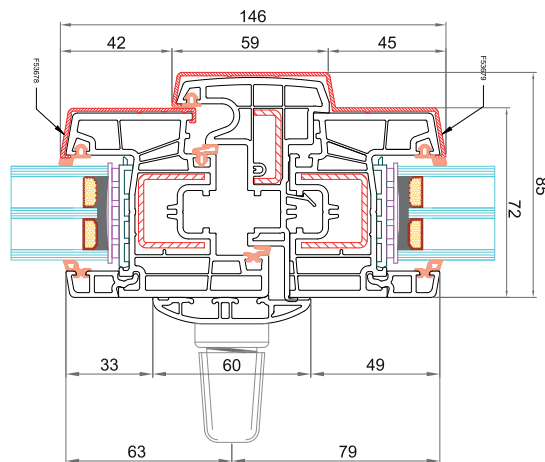
Anta CK-Z051 + AluClip F53678 Profilo di copertura arrotondato per maniglia centrale CK-E036 Battente mobile 58 mm CK-T046 Anta CK-Z051 + AluClip F53679
