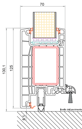
Anta CK-Z056 Barra parafreddo (nessuna soglia bassa)
