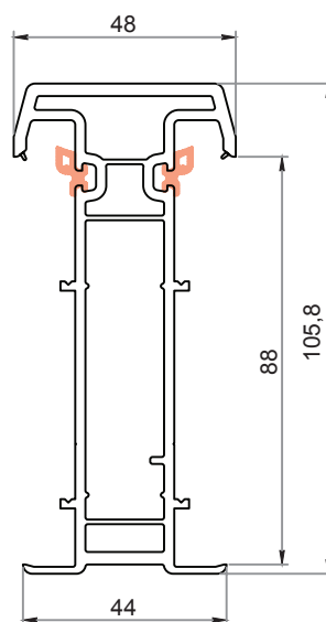
Connettore statico 28 mm 88605
