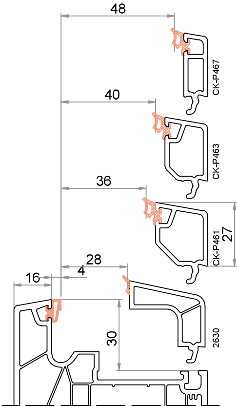
Telaio / Montante altezza della battuta 27 mm / altezza del fermavetro 27 mm
