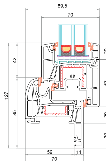
Telaio Reno 30 mm CK-L031 Anta CK-Z051
