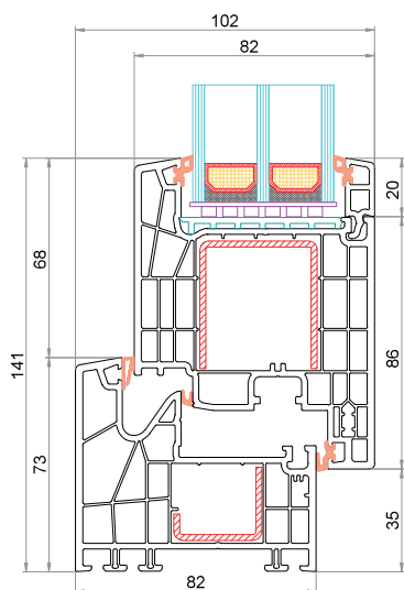
Telaio CK-L0802 Anta CK-Z841
