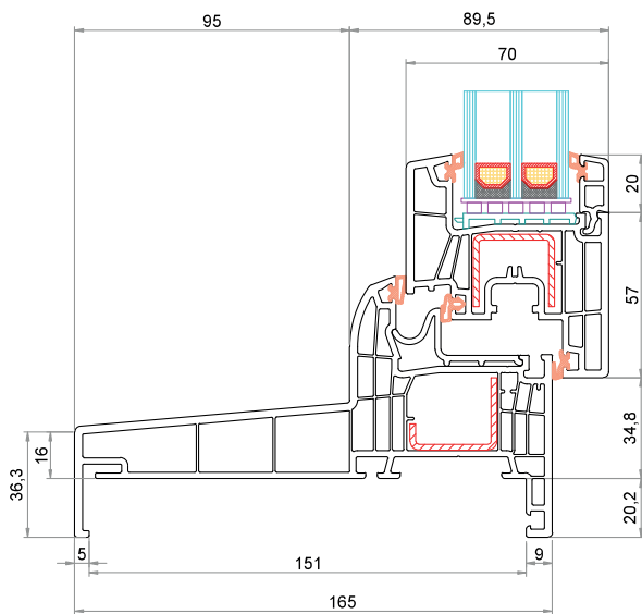
Telaio "Monoblocco" 165 mm CK-L028 Anta CK-Z051
