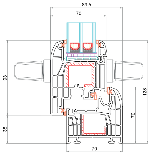
Telaio CK-L001 Anta CK-Z040 (maniglia passante)
